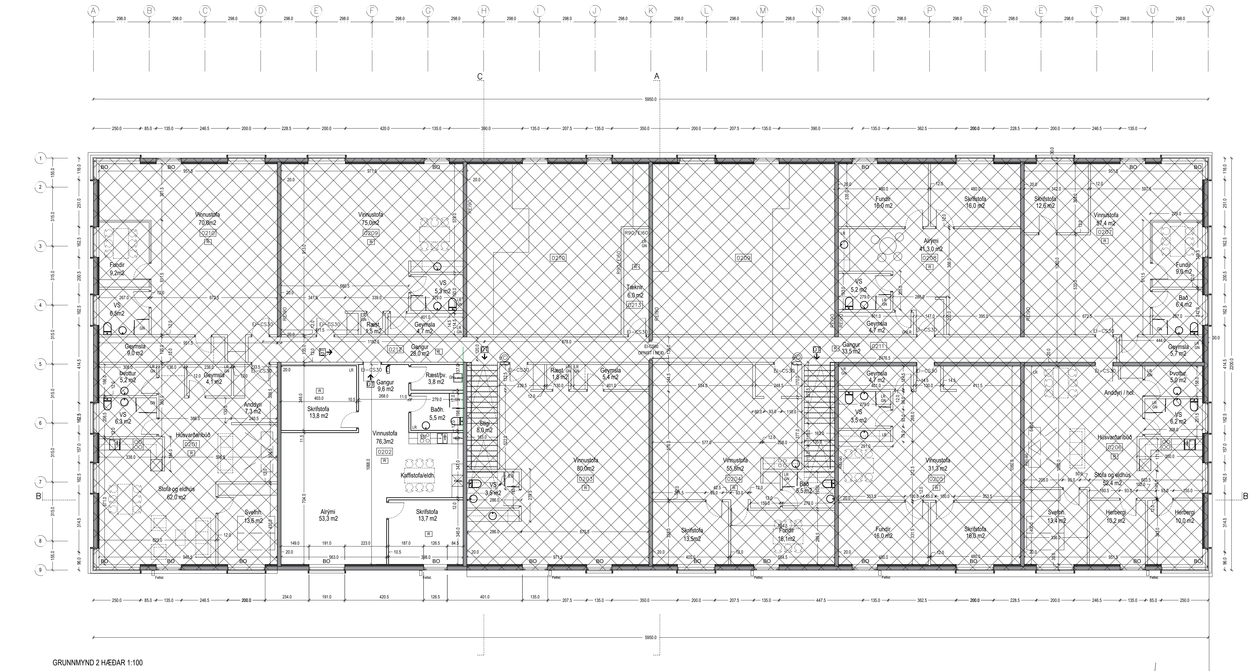
GRUNNMYND 2 HÆÐAR 1:100
